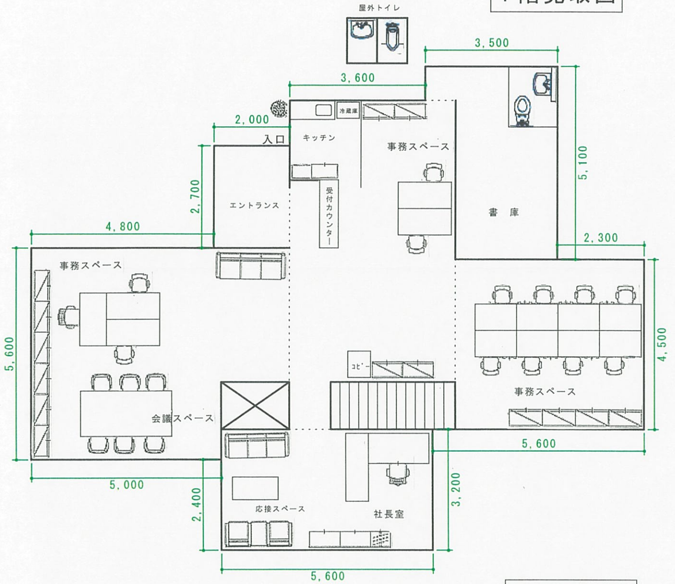
2階見取図
