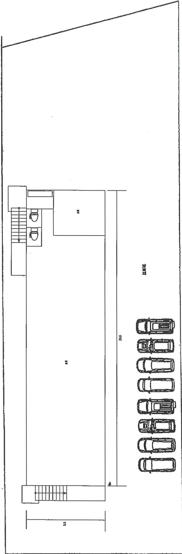
1階平面図
