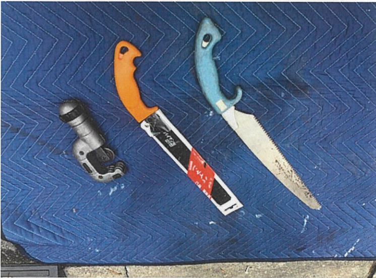
パイプカッター 塩ビのこ
