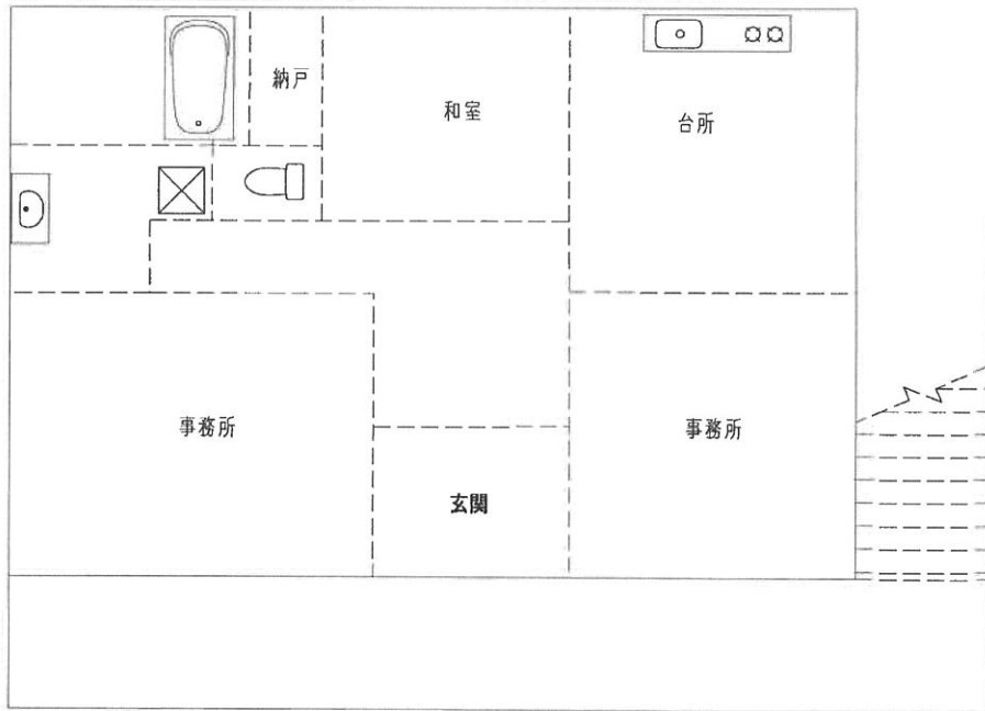
2階平面図
