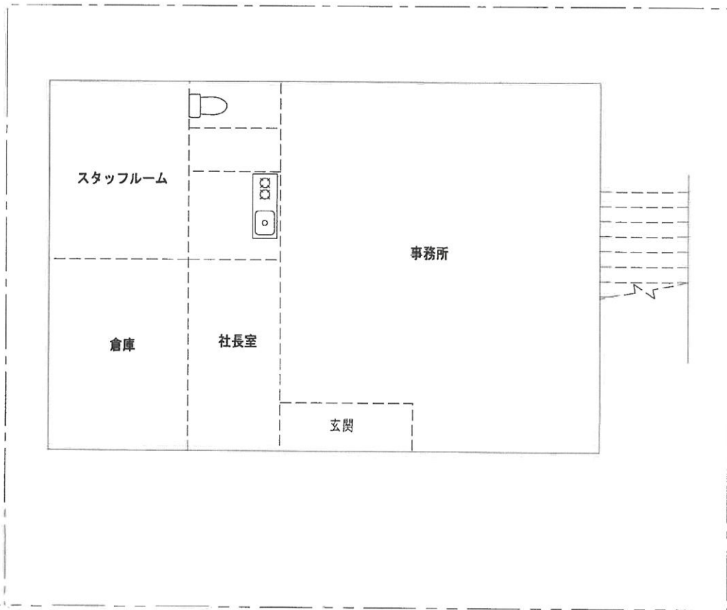
2階平面図
