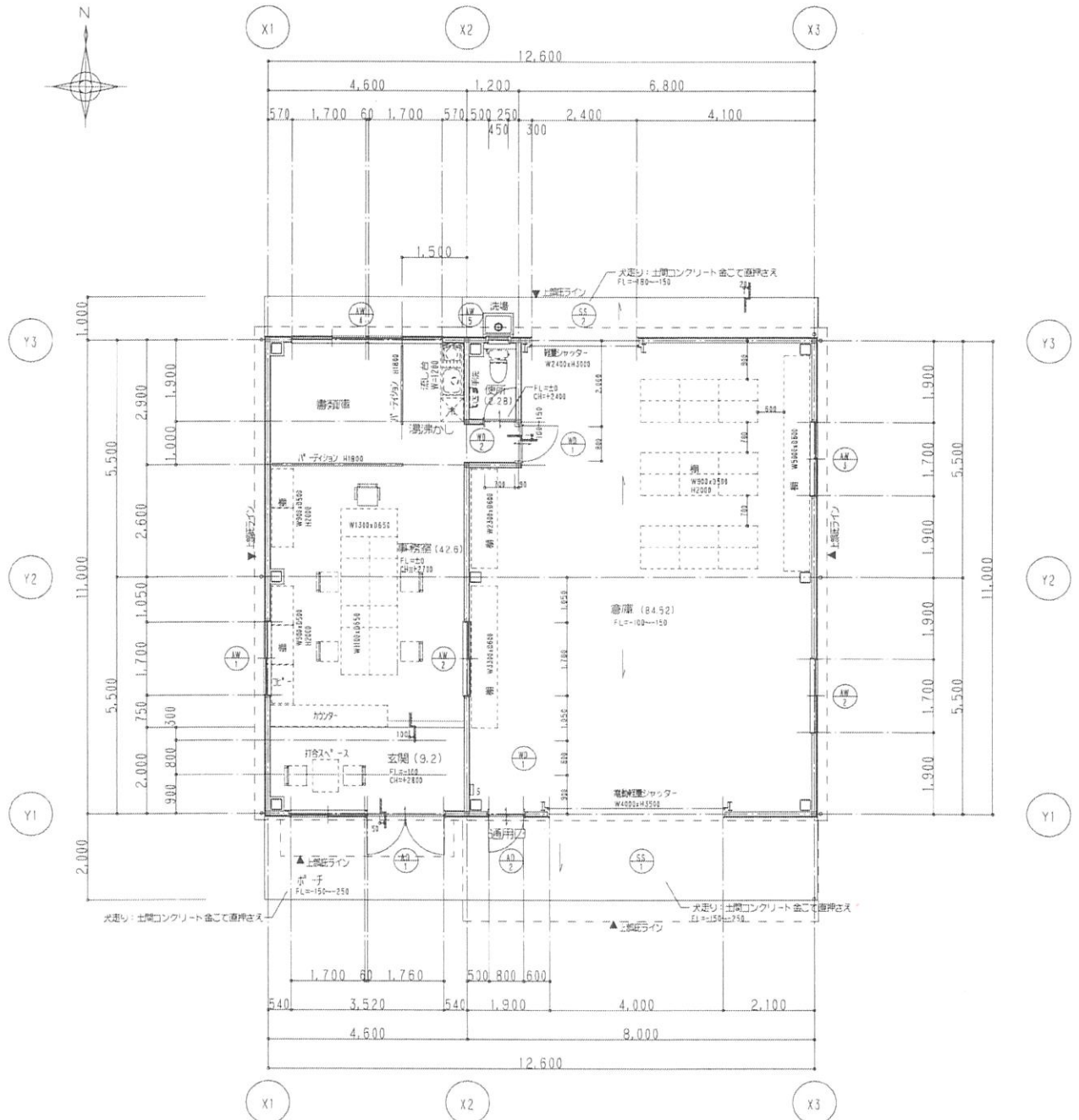
1階平面図 1:100
