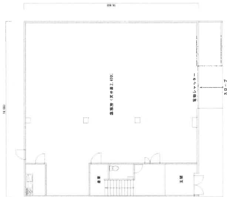
1階平面図
